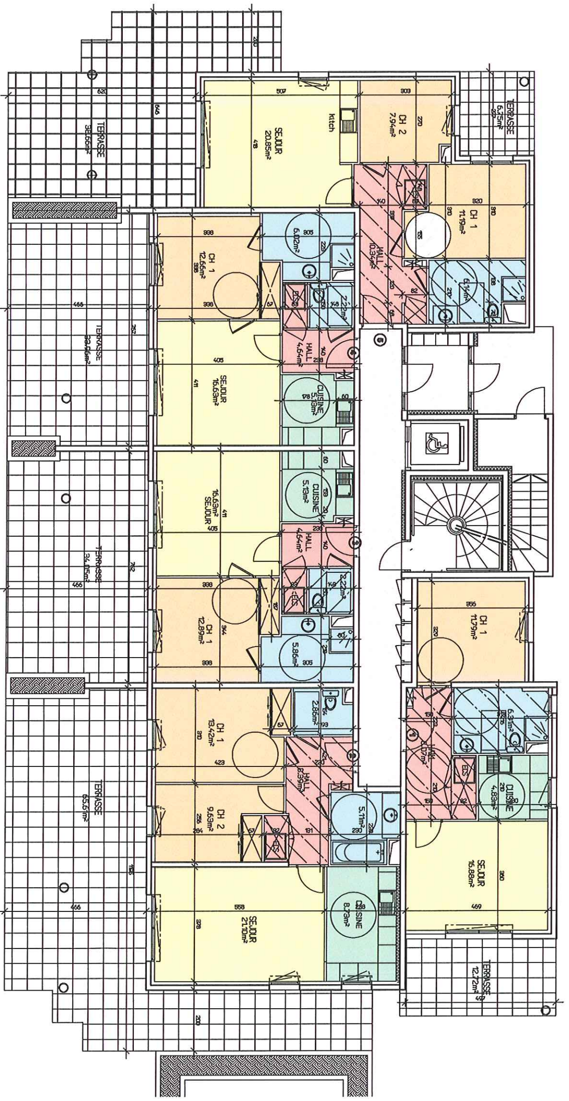
BATIMENT B - REZ DE CHAUSSEE
